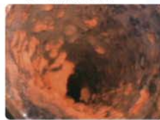
築50年の一般住宅の(水道管内をファイバースコープで撮影)例
